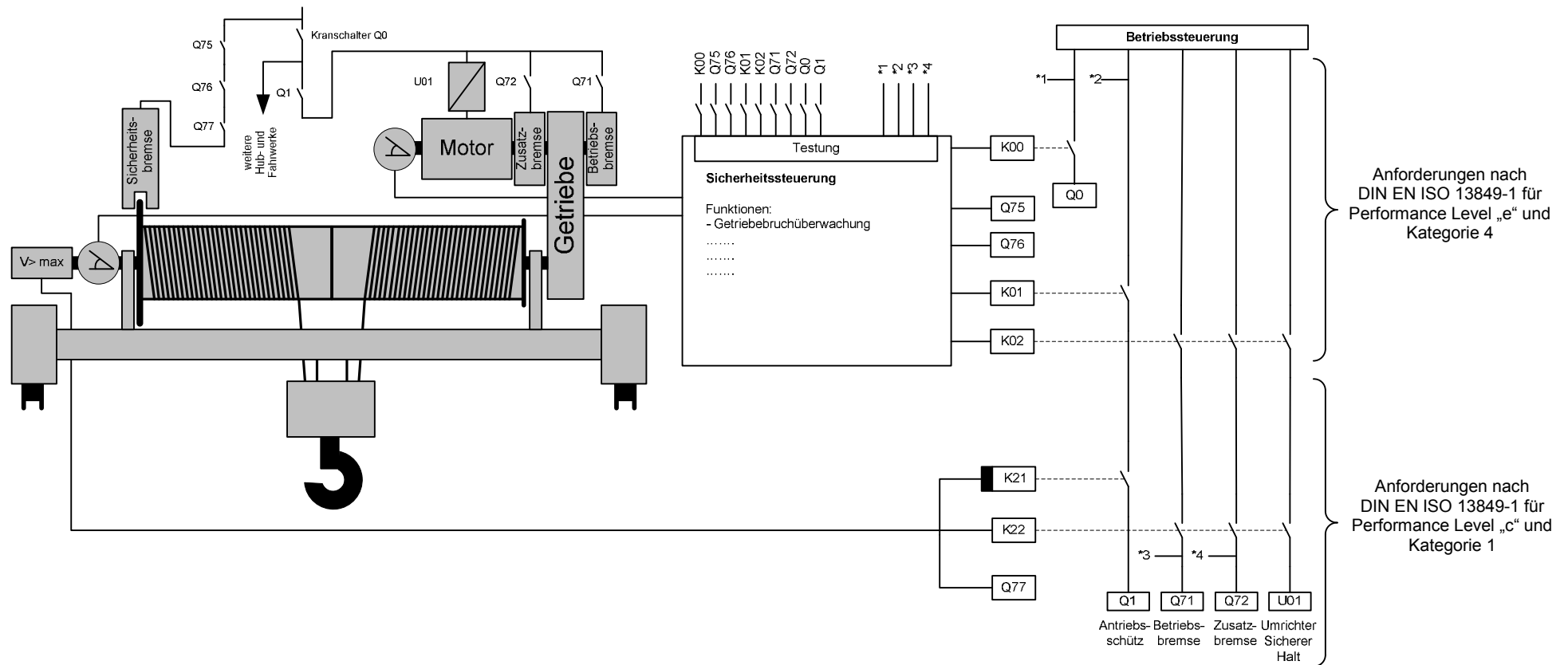
Bild E-2: Beispiel für eine Realisierung der Anforderungen gemäß Tabelle E-1 für die Funktion Ild. Nr. 31 „Getriebebruchüberwachung mit Ansteuerung der Sicherheitsbremse“ in Hebezeugen nach den Abschnitten 4.3 oder 4.4 (Beispiel für ein Hubwerk mit einfacher Triebwerkskette und Sicherheitsbremse)
