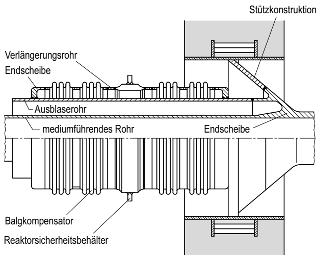
Bild 2-4: Bauteile von Rohrdurchführungen
