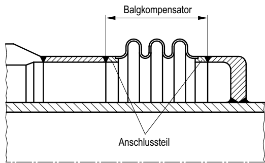
Bild 2-1: Anlussteil
