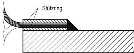
Bild 2-2: Stützring
