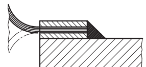
Einzelheit A Ausführungsform 4 für mehrlagige Bälge 2) 3)
