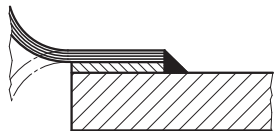
Einzelheit A Ausführungsform 5 für mehrlagige Bälge 2) 3)
