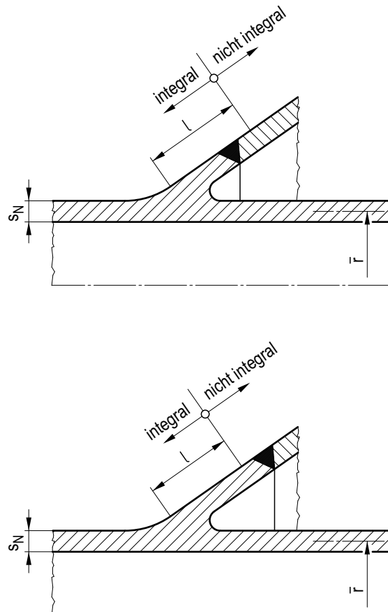
Bild 2-6: Beispiele für Stützkonstruktionen
