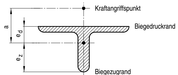
Bild A-3: Stabquerschnitt mit e_z > e_d
