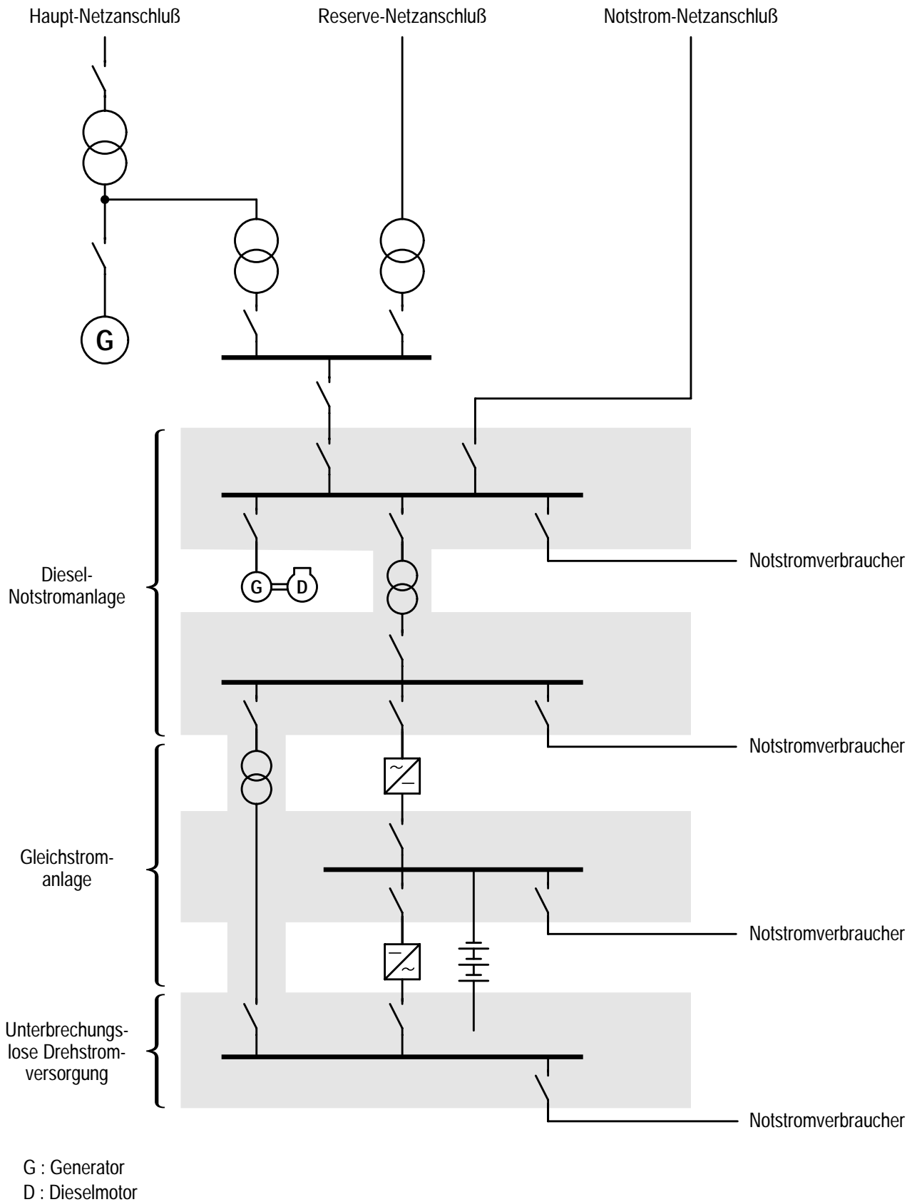
Bild 1-1: Grenzen der Regel KTA 3705
