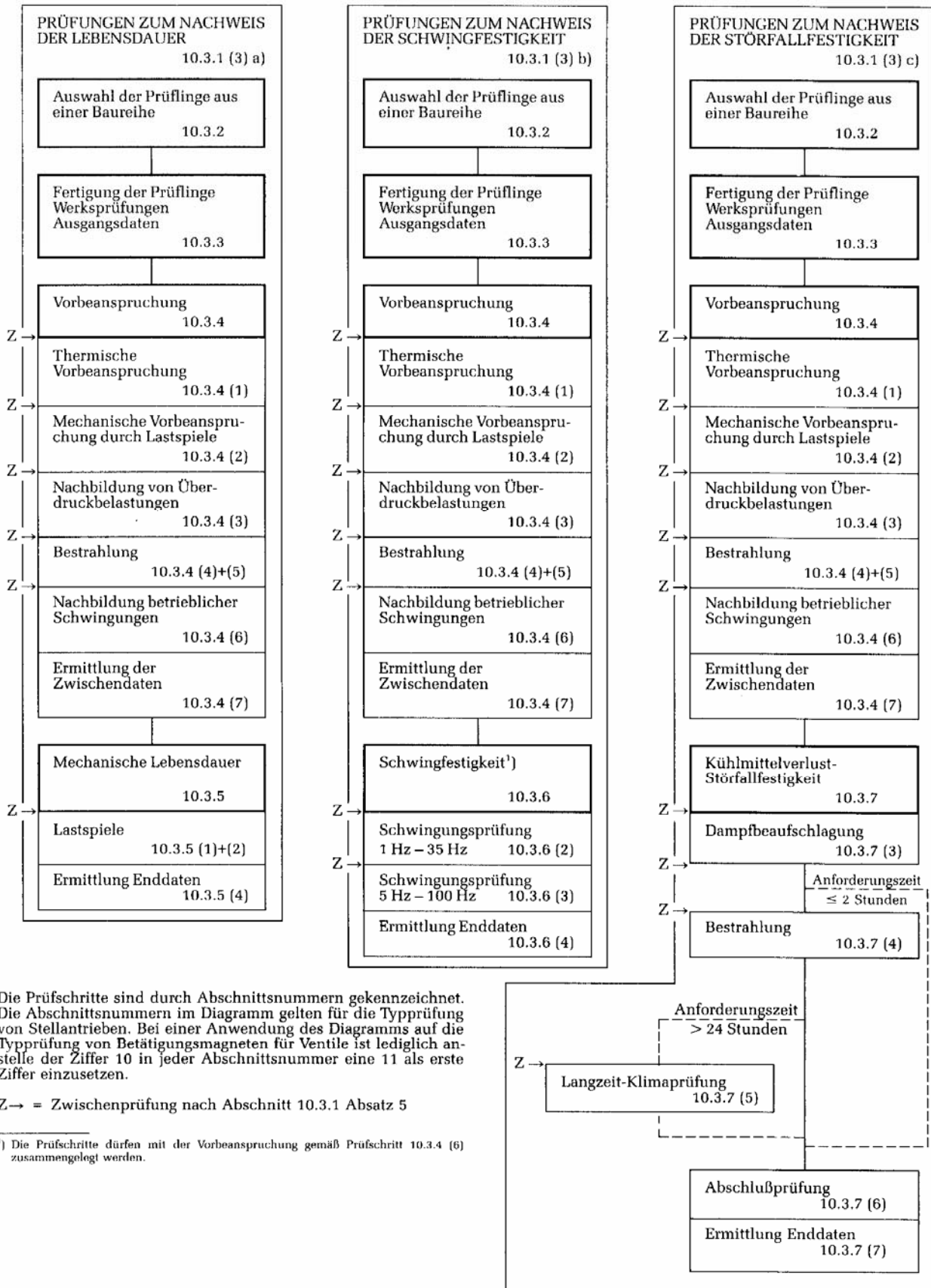
Bild 10-1: Prüfschritte der praktischen Typprüfungen für eine Baureihe von Stellantrieben nach Abschnitt 10 oder eine Baureihe von Betätigungsmagneten für Ventile nach Abschnitt 11
