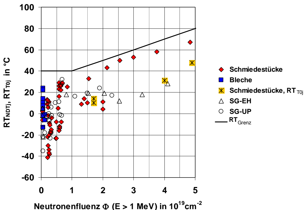
Bild B-1: RT_{\text{NDTj}} , RT_{\text{Toj}} als Funktion der Neutronenfluss, Grundwerkstoff- und Schweißgüterergebnisse der Bestrahlungsüberwachungsprogramme der deutschen RDB (SWR und DWR); nur Schweißgüter mit Massenanteilen \text{Cu} \leq 0,15 \% und 0,05 \% < \text{Ni} \leq 1,7 \% .
