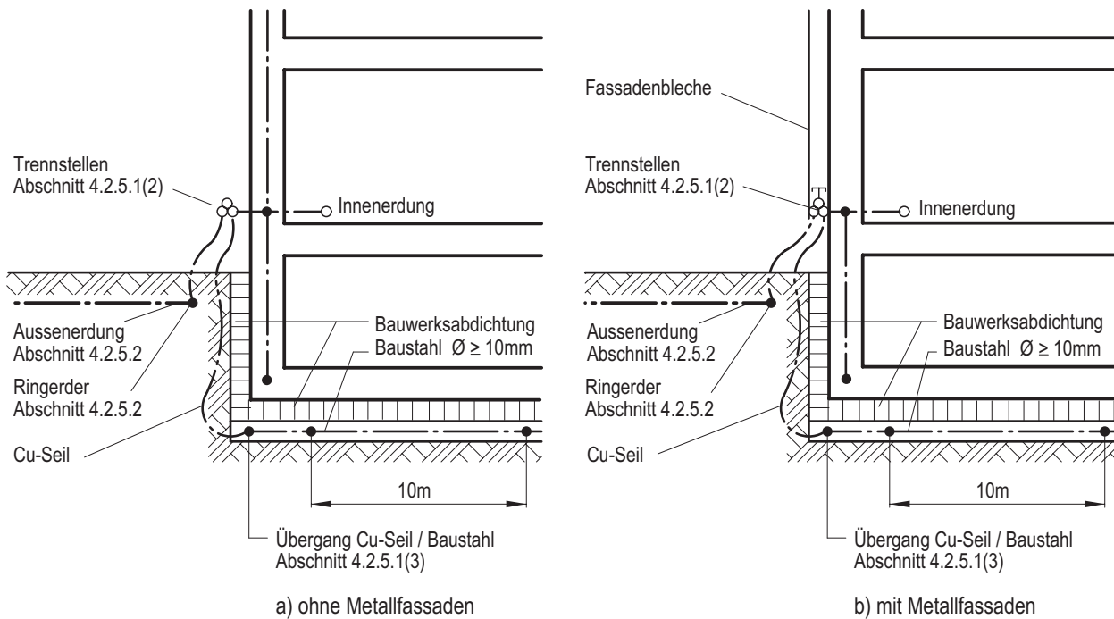
Bild 4-2: Anschluss des Fundamenterders bei Gebäuden mit außen liegender Bauwerksabdichtung
