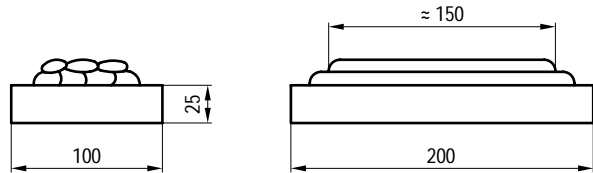
Bild 4.7.2-1: Prüfstück für Schweißpanzerungen
