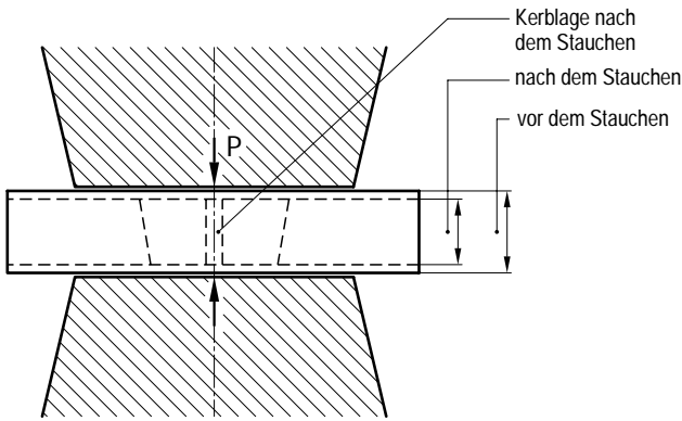
Bild 4.5.5-1 Stauchen von zu alternden Kerbschlagbiegeproben
