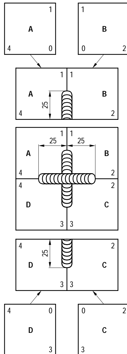
Bild E-2: Vorbereiten des Prüfstückes
